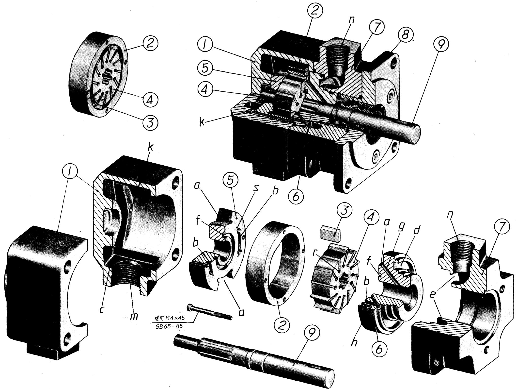
图 1—4 YB 1 -25 型叶片泵轴测图
