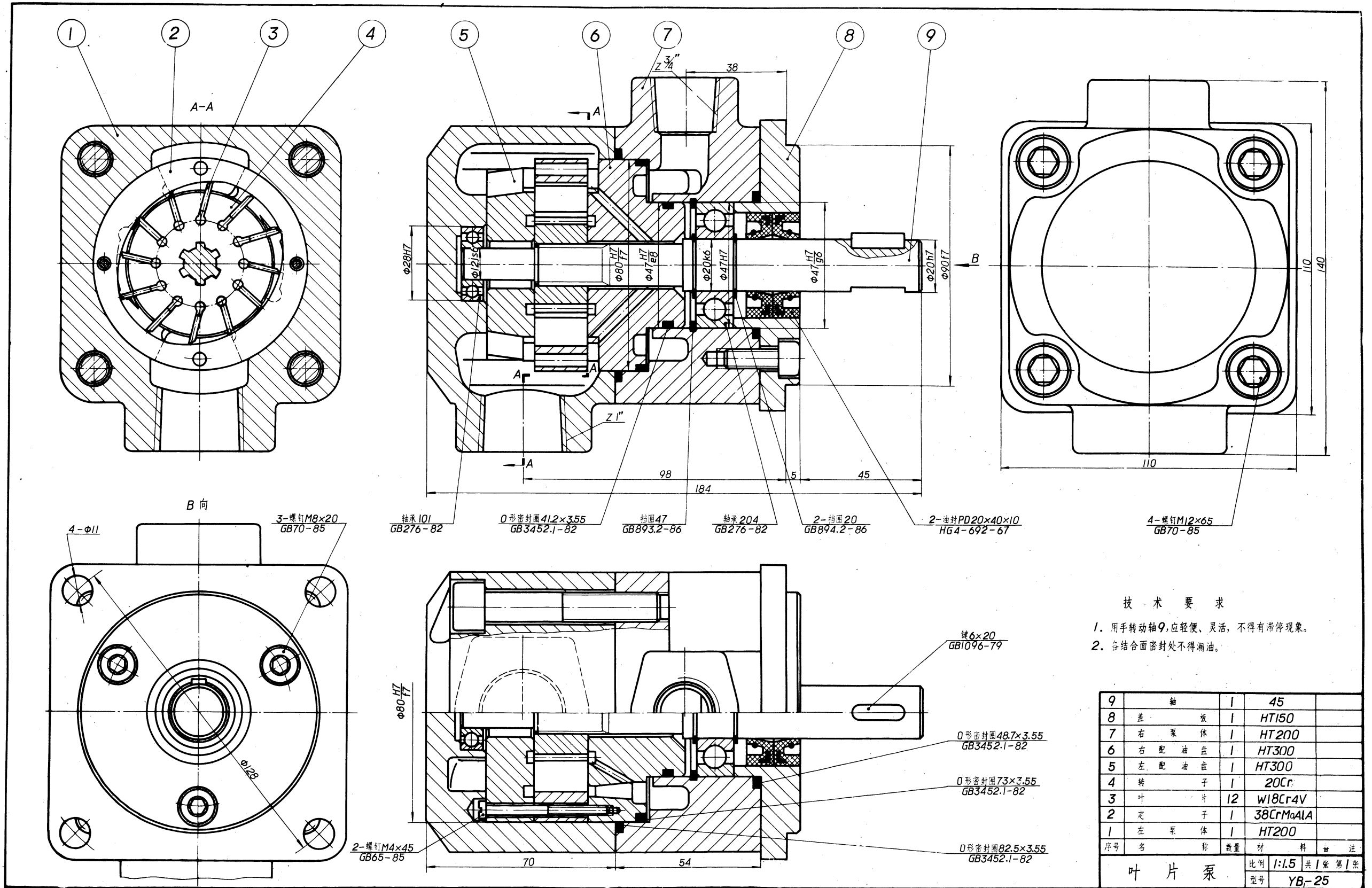
图 1-3 YB 1 -25 型叶片泵装配图
