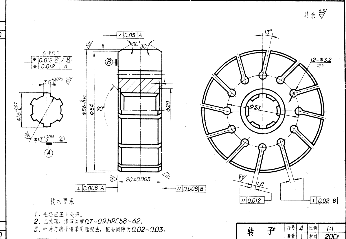
图 1—5 YB 1 -25 型叶片泵零件图(一)
