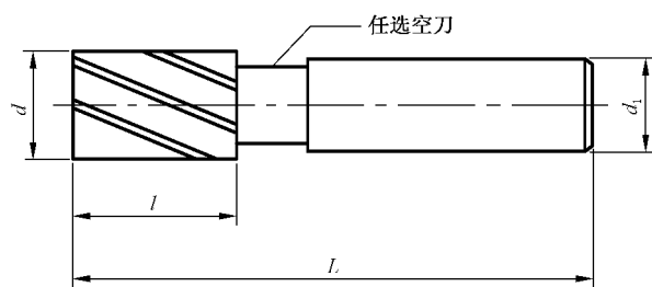
图 1 普通直柄立铣刀
