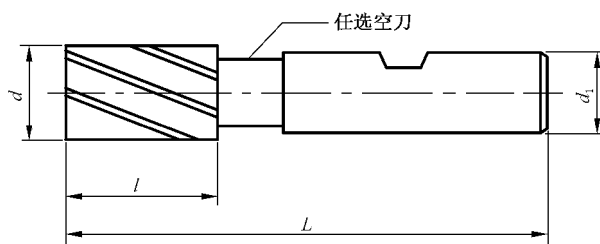
图 2 削平直柄立铣刀
