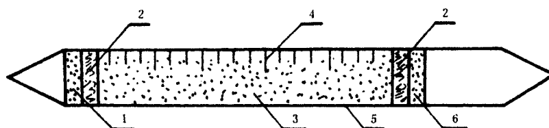
图 1 比长式硫化氢检测管示意图
