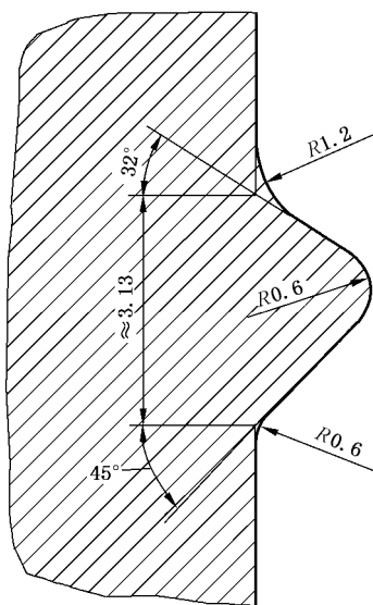
图 1 铣刀轮廓
