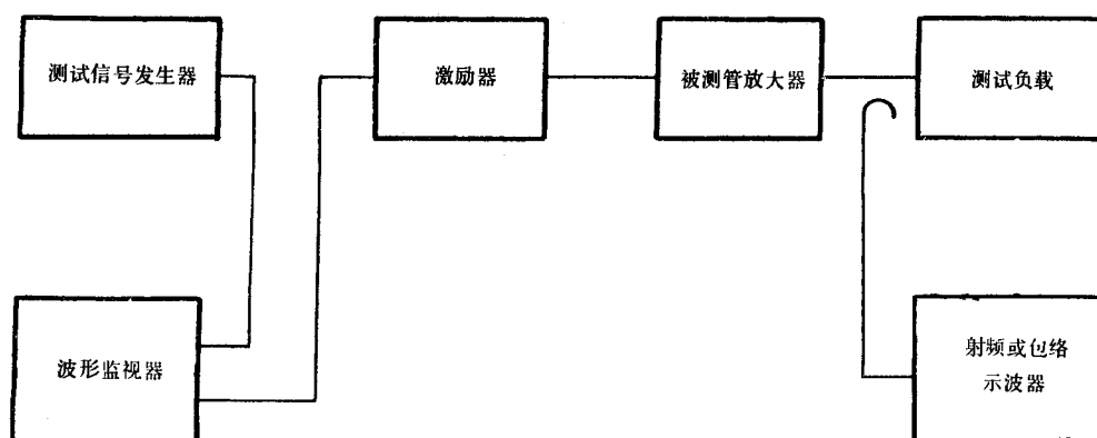
图 1 同步脉冲压缩测试方框图
