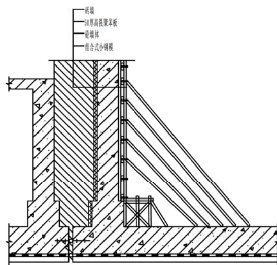
①-③处沉降缝施工示意图
