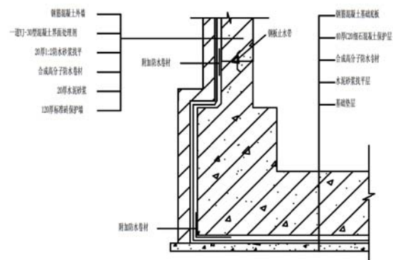
底板及地下室外墙防水做法图3
