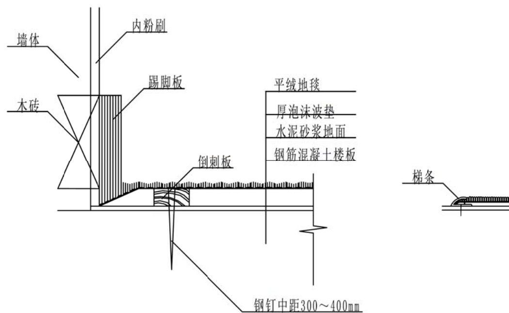
倒刺板及梯条图
