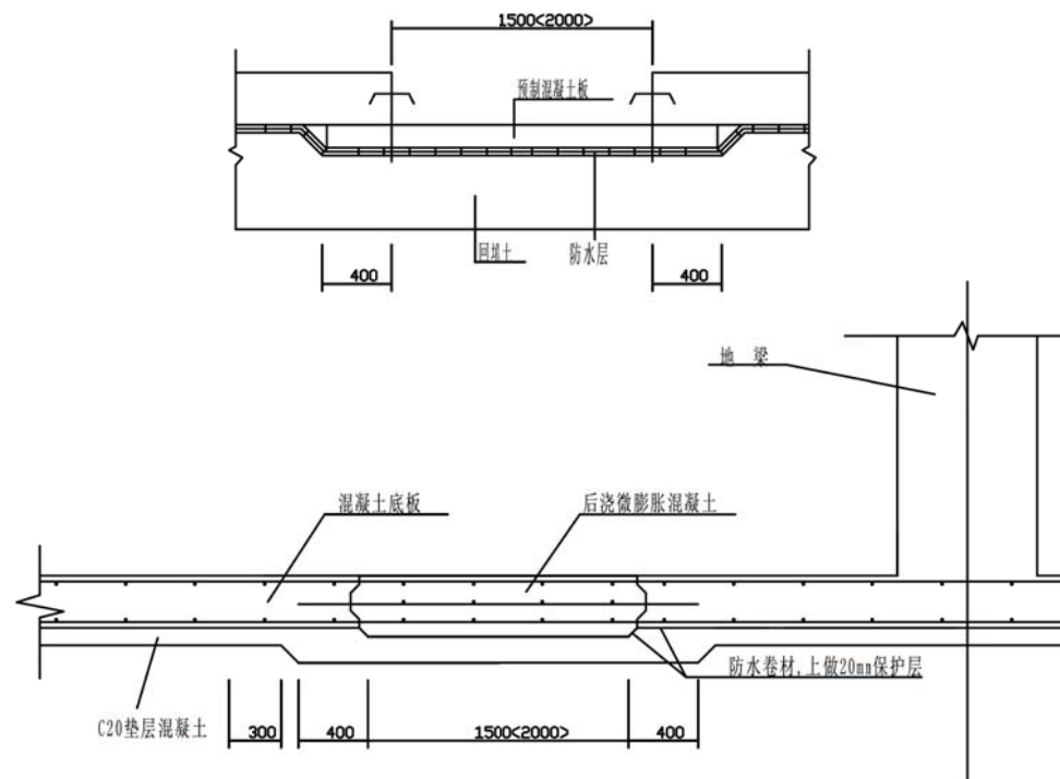
地下室底板后浇带处理构造图2
