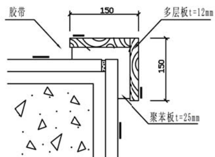
石材转角的保护方法
