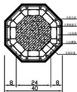
独立柱石材安装示意图
