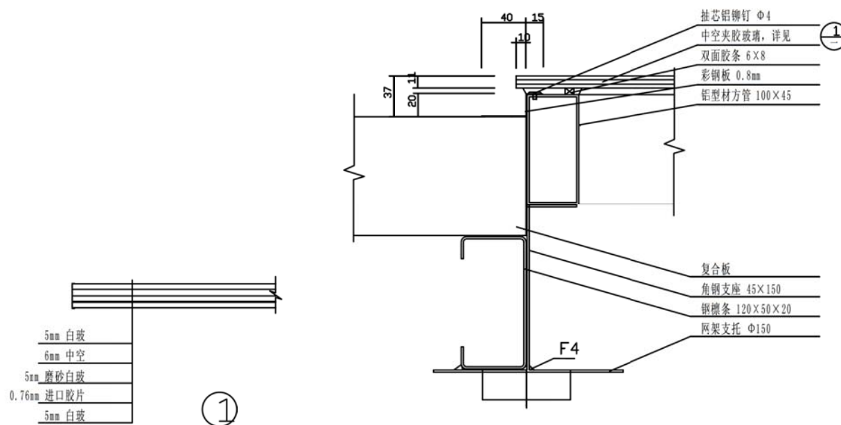
玻璃采光顶与彩钢复合板结点详图
