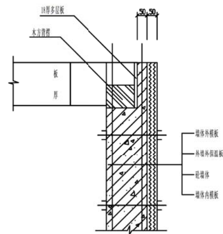
外墙楼层接缝示意图
