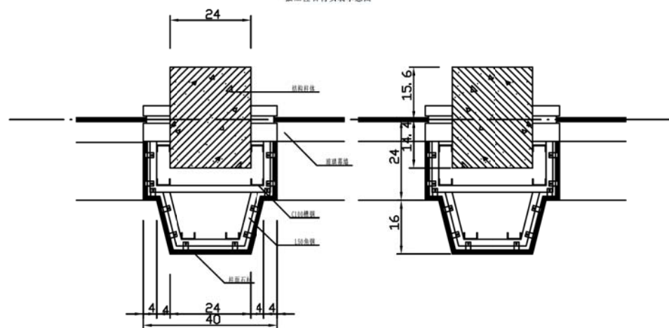
窗侧柱身石材安装示意图
