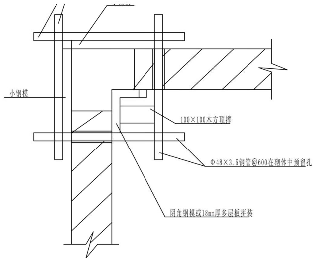
"L"型墙转角处构造柱支模示意图
