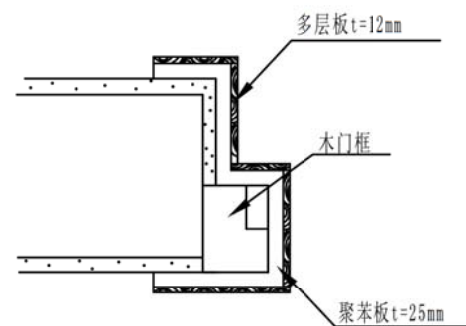
装修完成后的木门框保护
