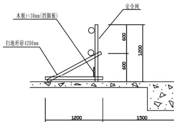
1. 临边防护 (适用于建筑周边、中庭)
