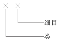
图 1 代码结构图
