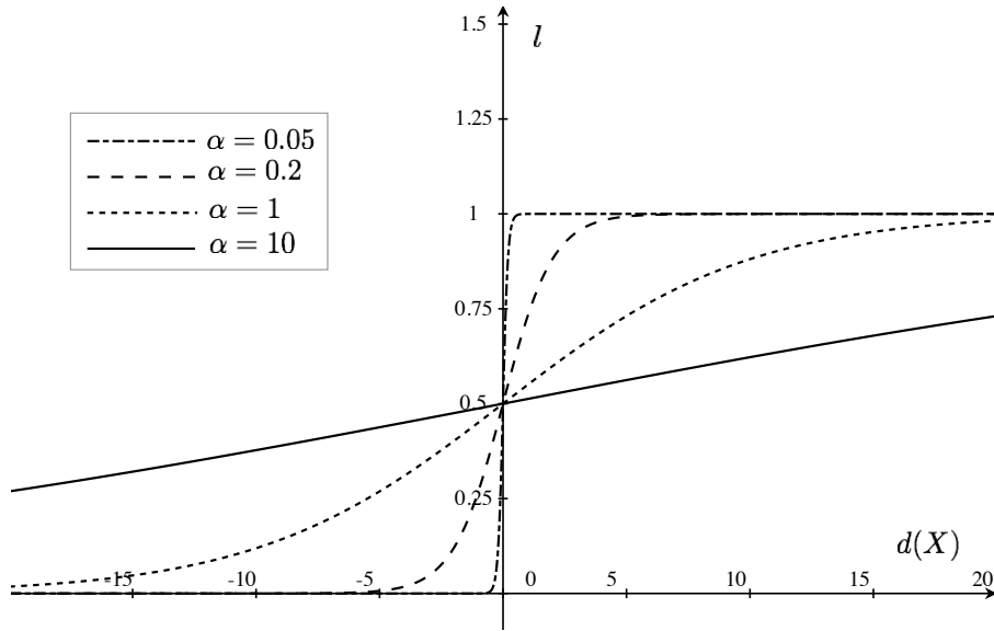
图5.1 目标函数随 \alpha 变化示意图
