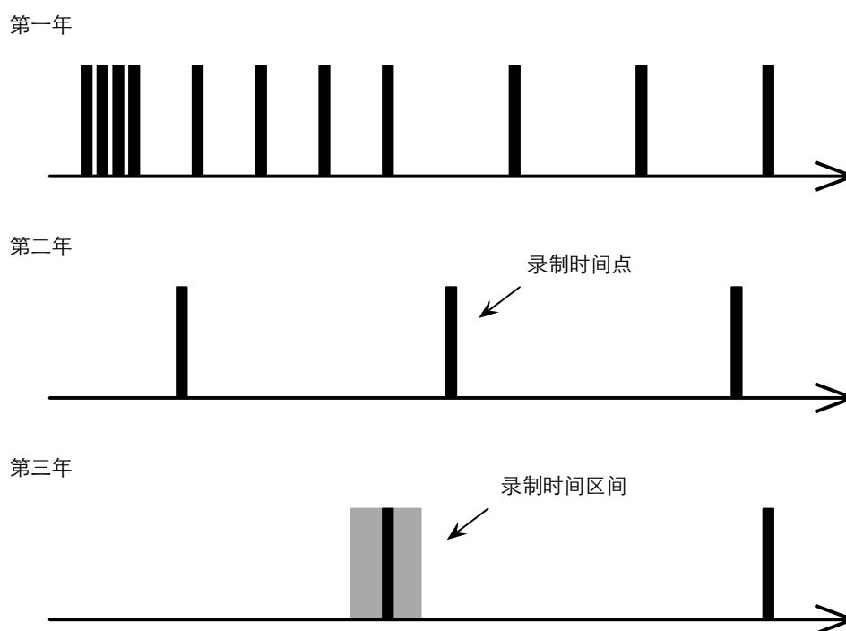
图2.2 Chronos录制时间间隔设计
