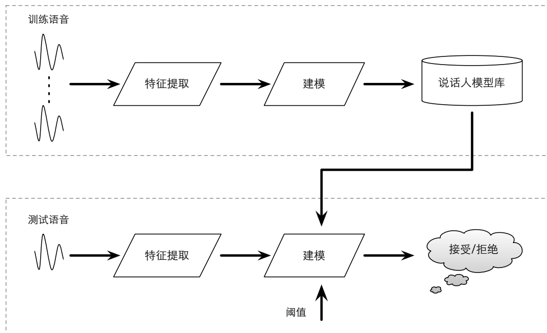
图 1.1 一个典型的说话人确认系统框架
