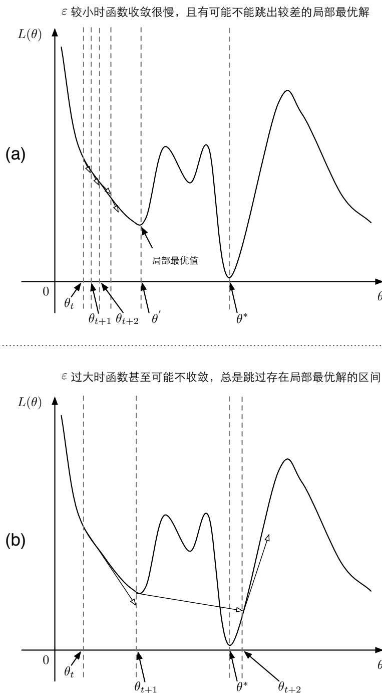
图5.2 搜索步长的影响示意图
