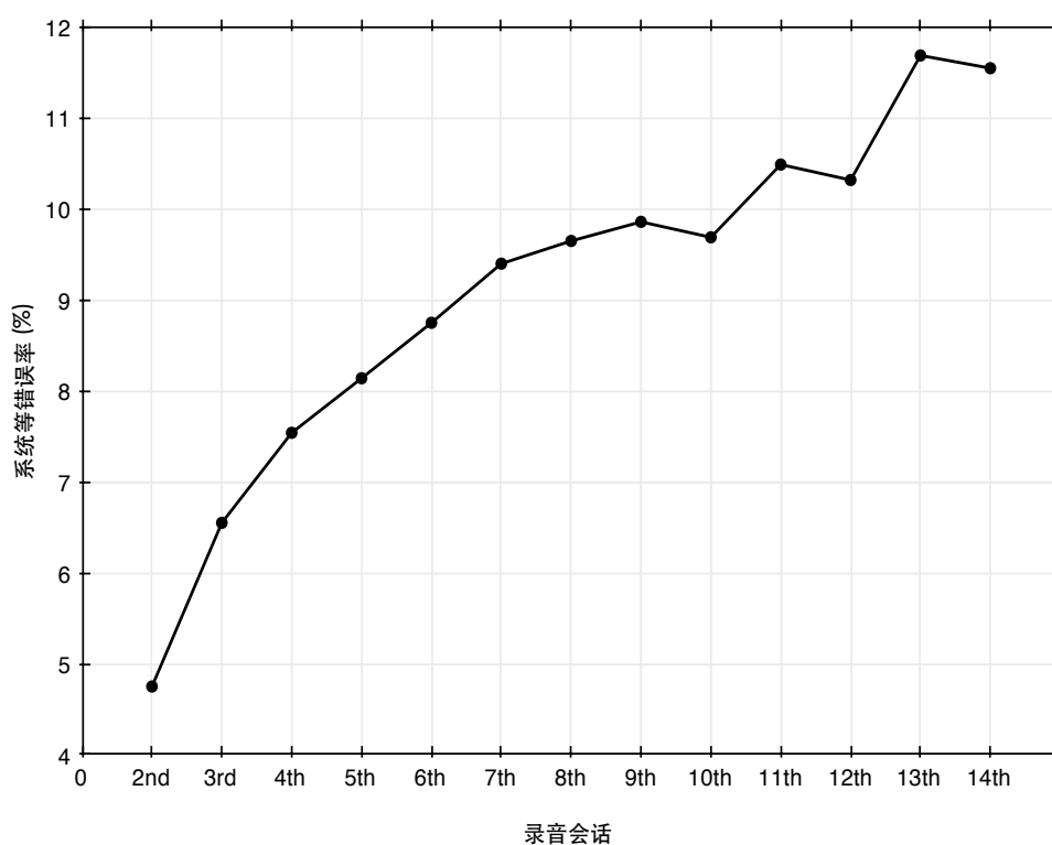
图2.6 不同录音会话的等错误率变化曲线（训练数据来自第二次）
