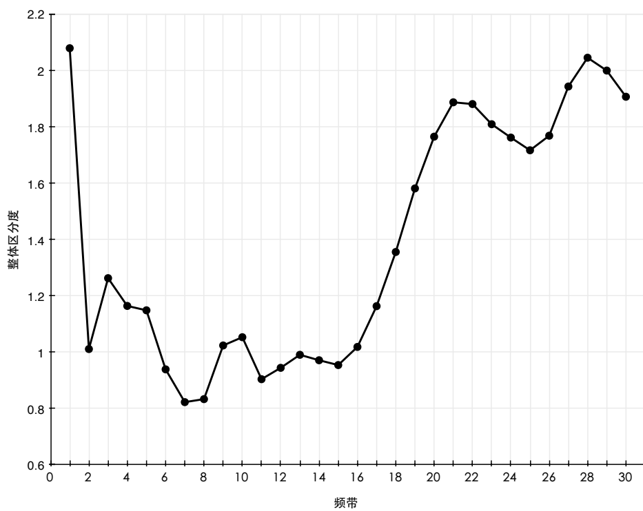
图3.8 以基于频带能量的F-ratio为中间准则计算得到的频带整体区分度曲线
