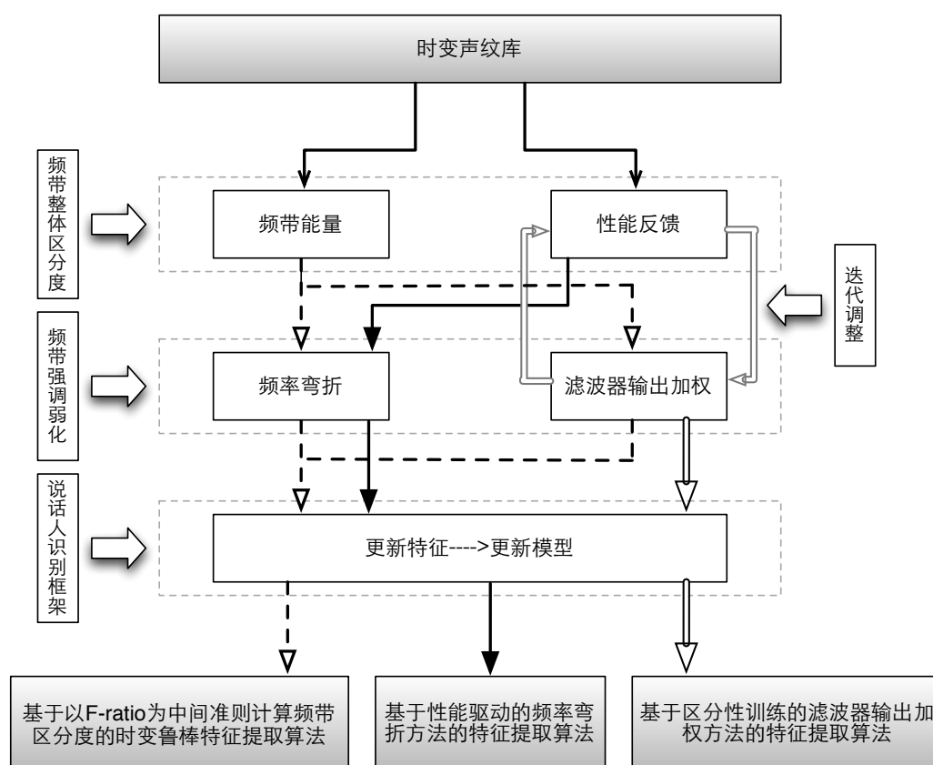
图1.5 论文工作内容示意图
