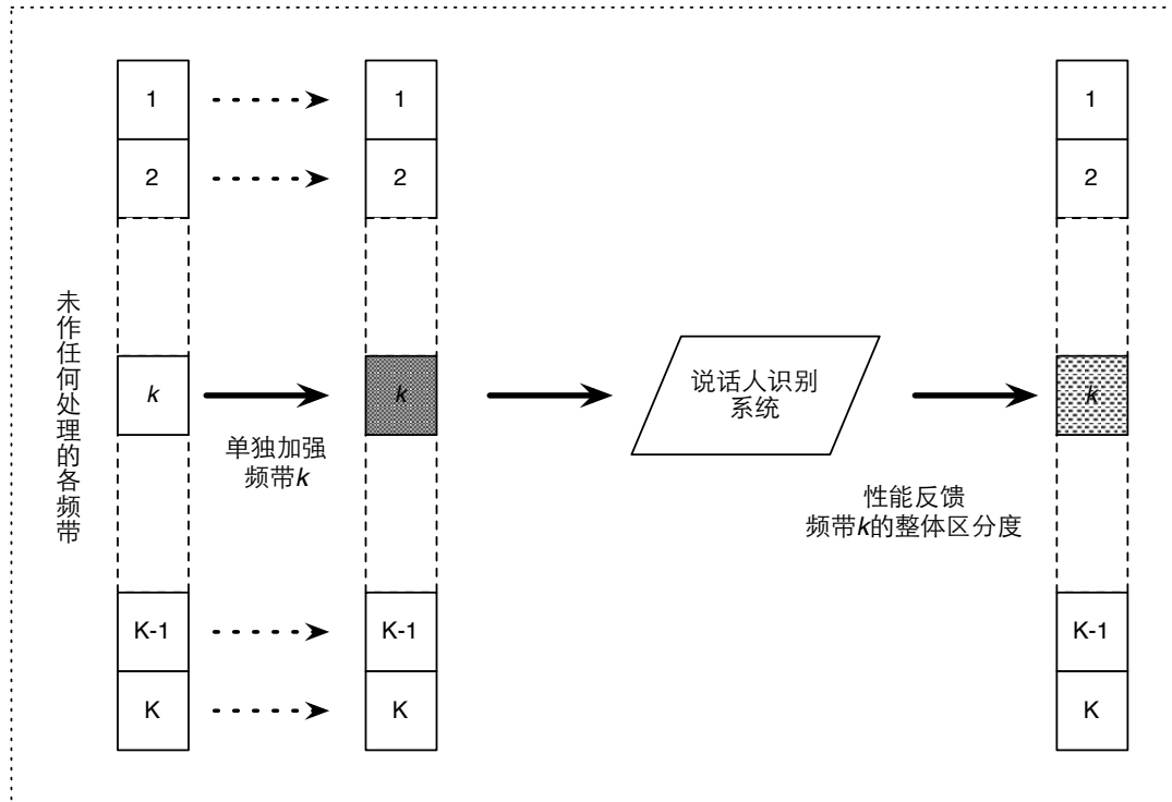
图 4.1 性能驱动准则的总体框架示意图
