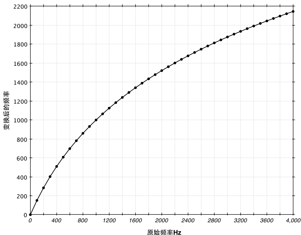
图1.4 MFCC的频率弯折示意图
