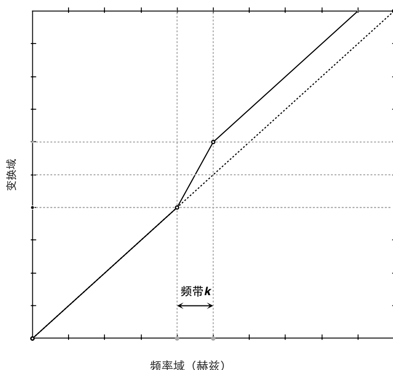
图4.2 单独加强频带 k （两倍时）的频率弯折示意图
