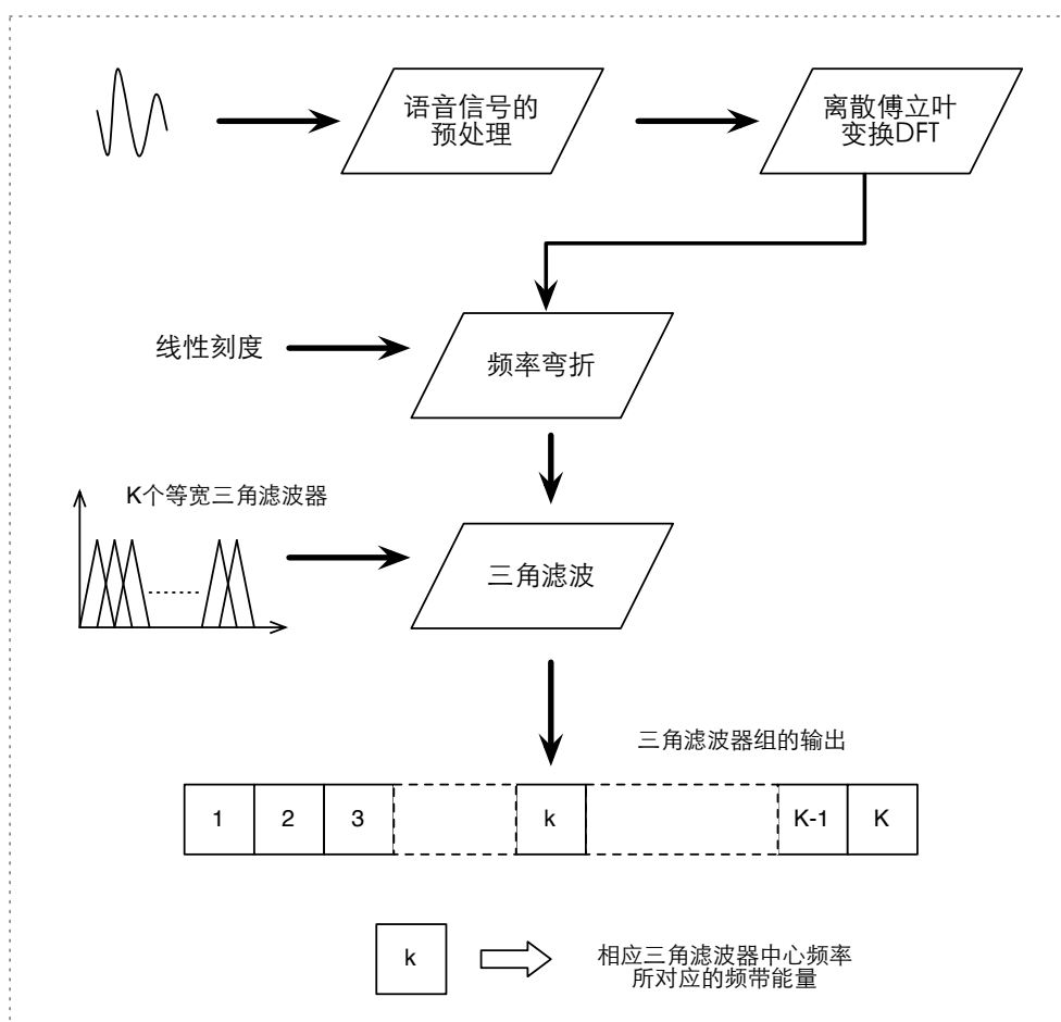
图3.2 频带能量参数计算过程示意图
