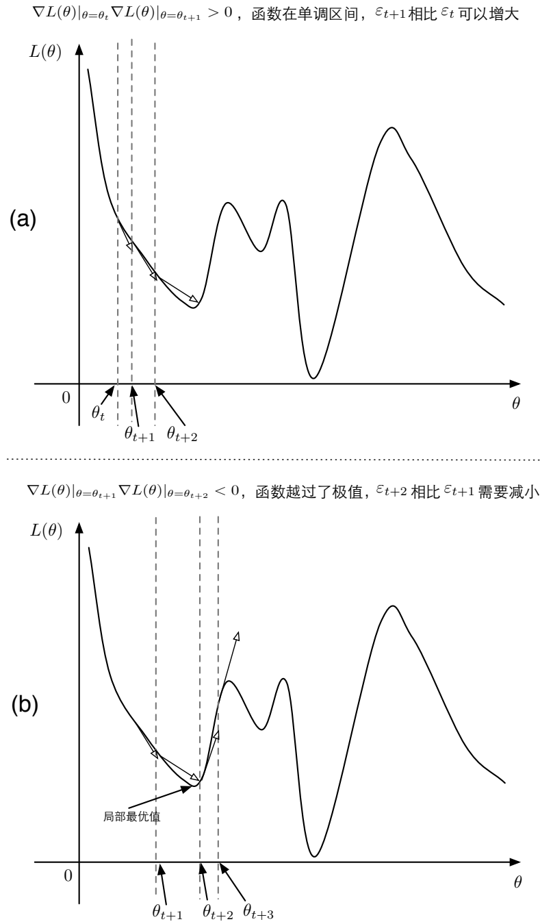
图5.3 RProp算法搜索步长弹性变化示意图
