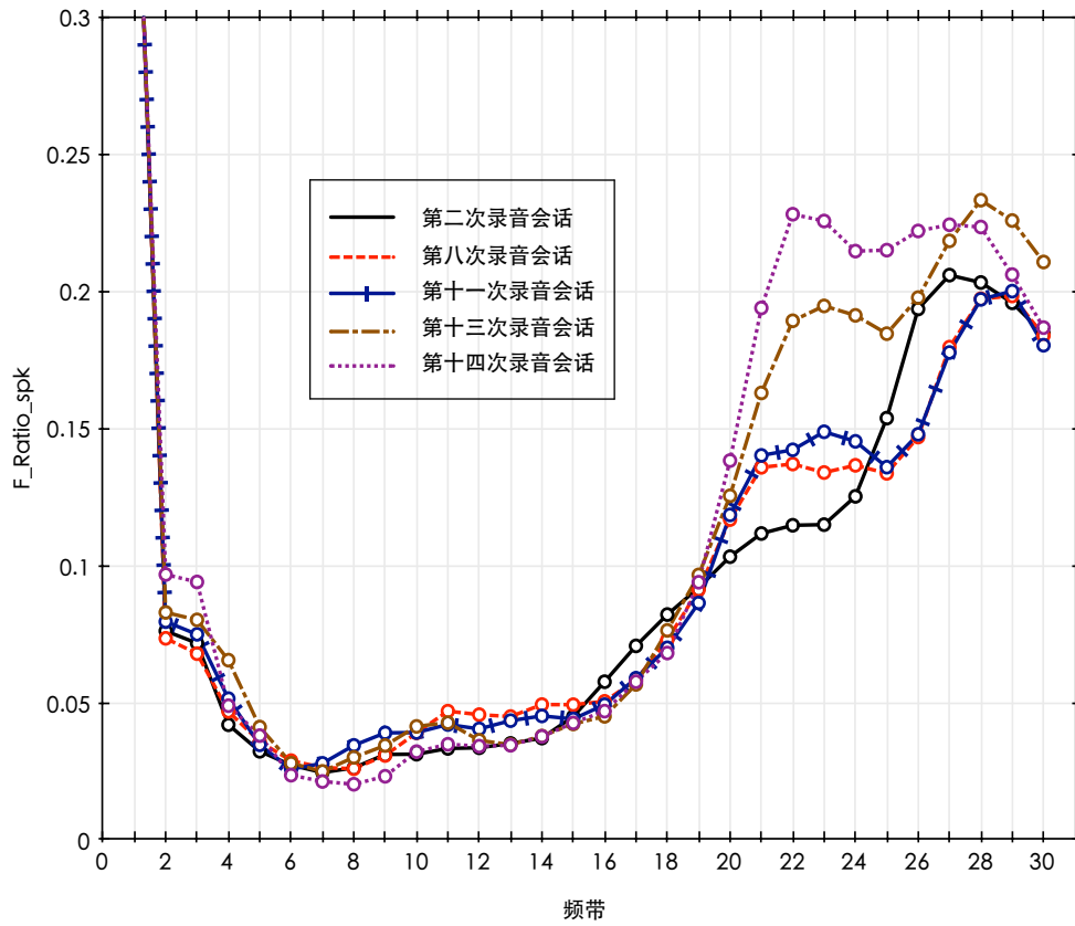
图3.6 间隔大约半年的五次录音会话的对应说话人个性信息区分度曲线示意图
