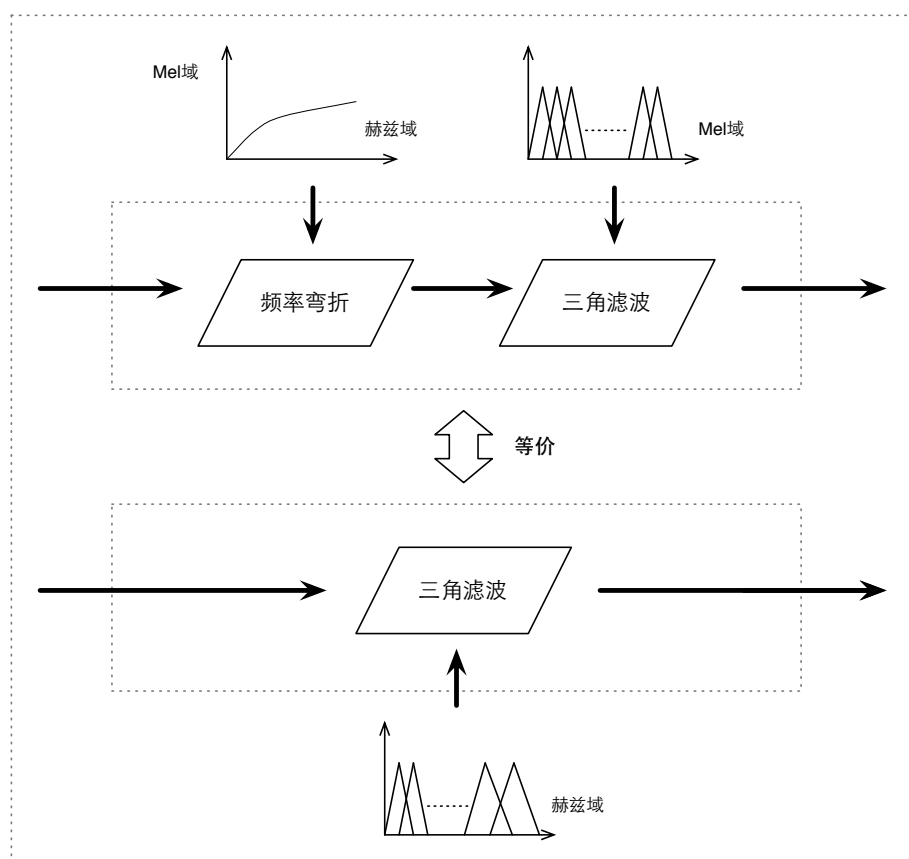
图3.3 提取MFCC特征时Mel域和赫兹域的三角滤波器组设置示意图
