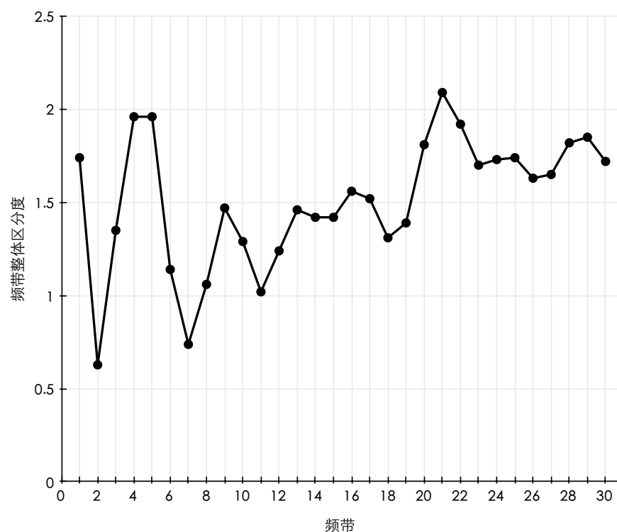
图5.4 MCE*MSV准则下的滤波器输出权重折线图
