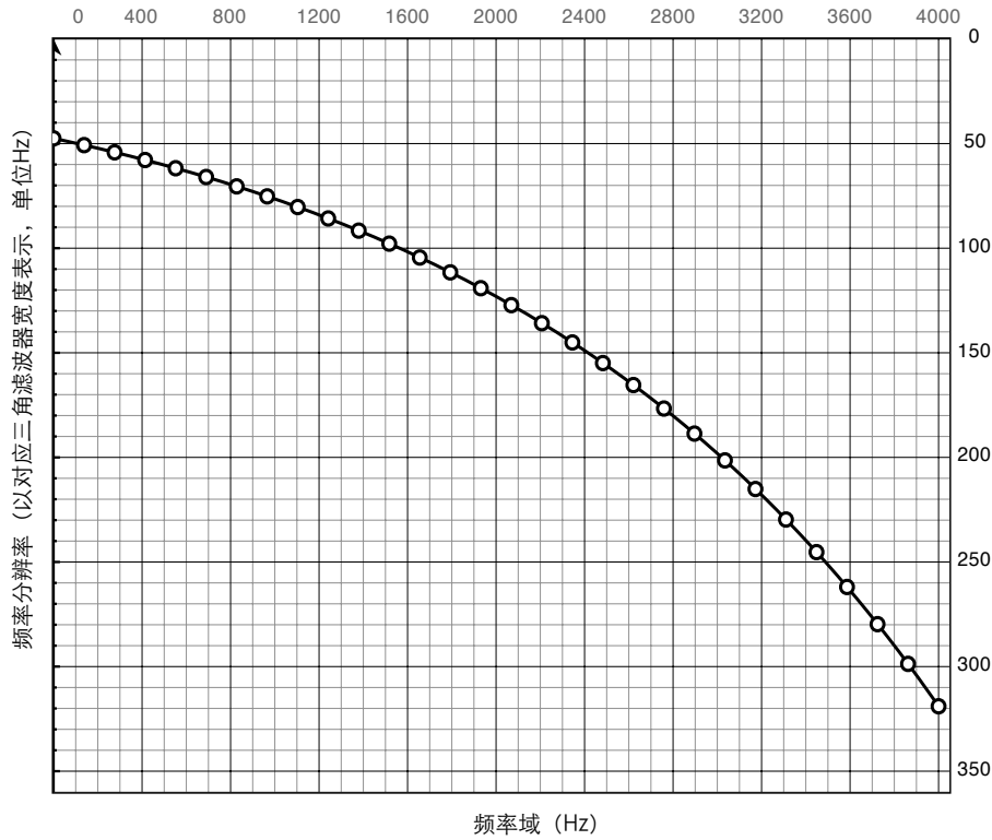
图3.4 MFCC特征提取时不同频带的分辨率
