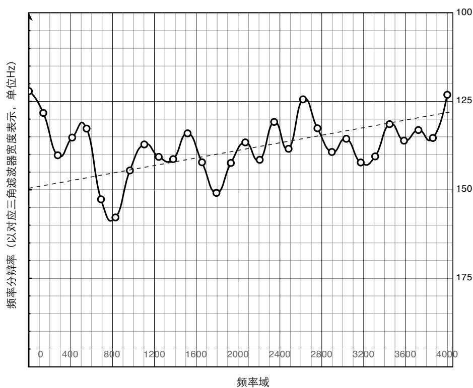
图4.3 性能驱动准则下的频带分辨率（Hz）
