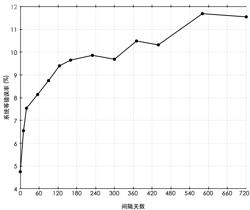
图 2.7 不同录音会话的等错误率变化曲线（以间隔天数作为横轴）
