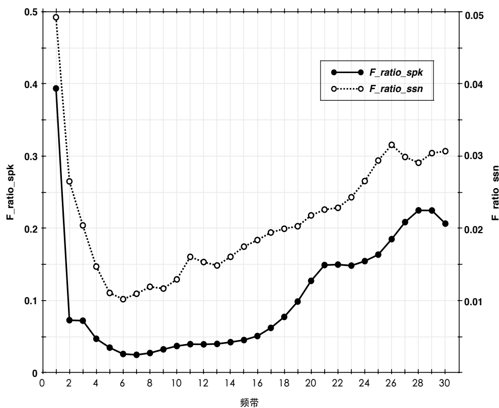
图3.7 两种区分度 ( F\_ratio\_spk 和 F\_ratio\_ssn ) 曲线示意图
