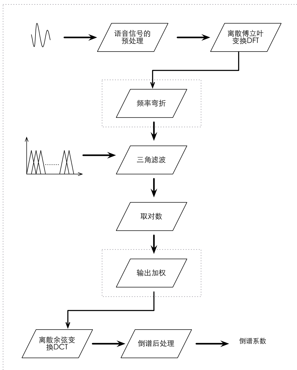
图1.3 倒谱系数计算流程示意图
