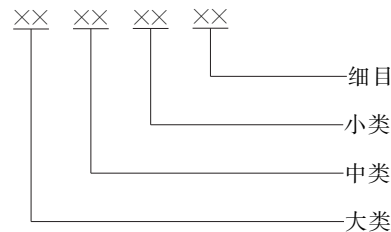
图 1 代码结构图
