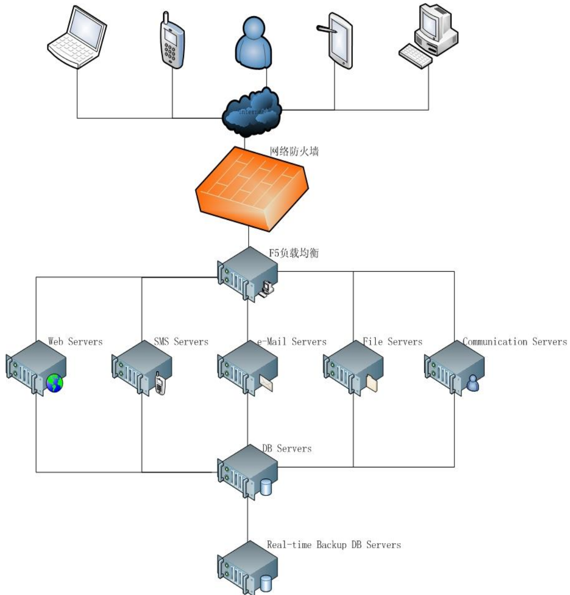
图 3.1 系统架构图
