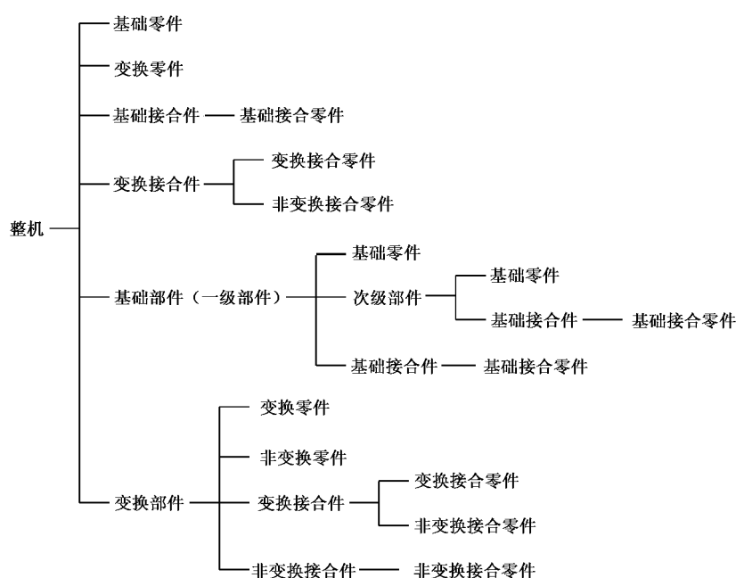
图 1 产品专用件分类及其隶属关系
