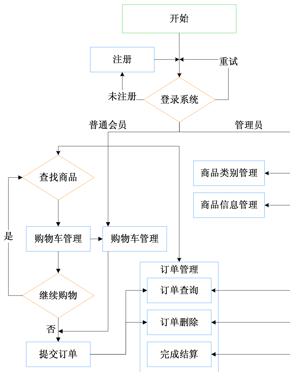
图 4.5 系统主要业务流程
