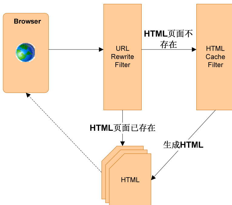
图 5.11 自动生成静态 HTML 机制
