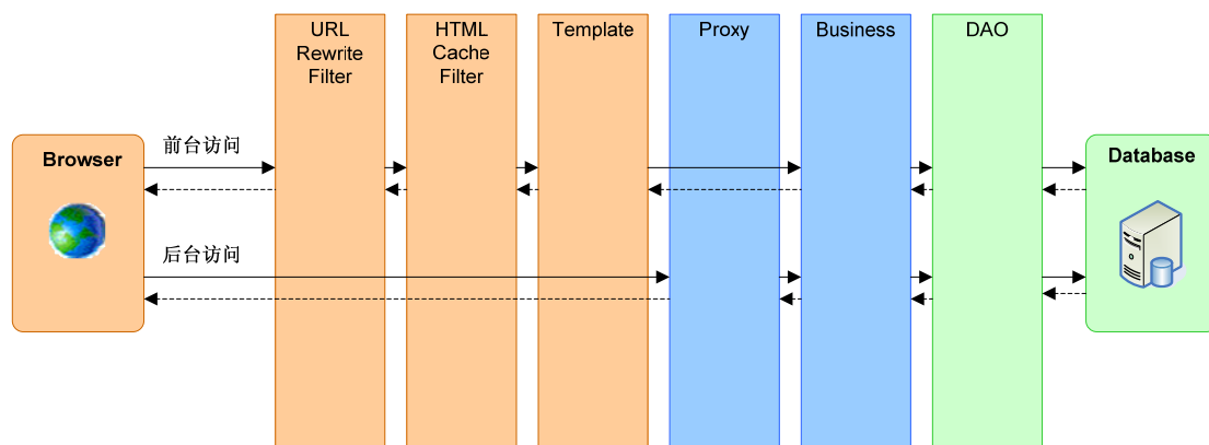
图 4.3 页面请求数据流程
