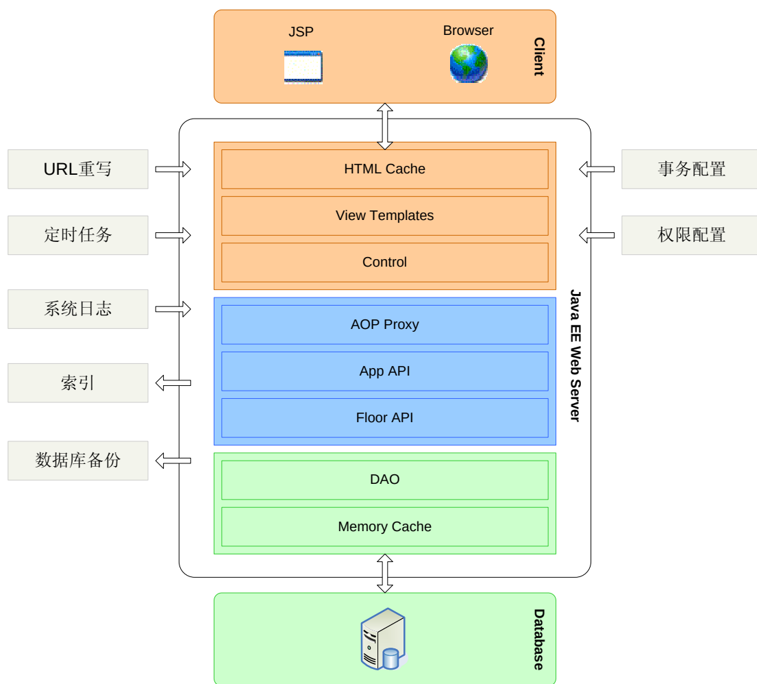
图 4.2 系统逻辑架构
