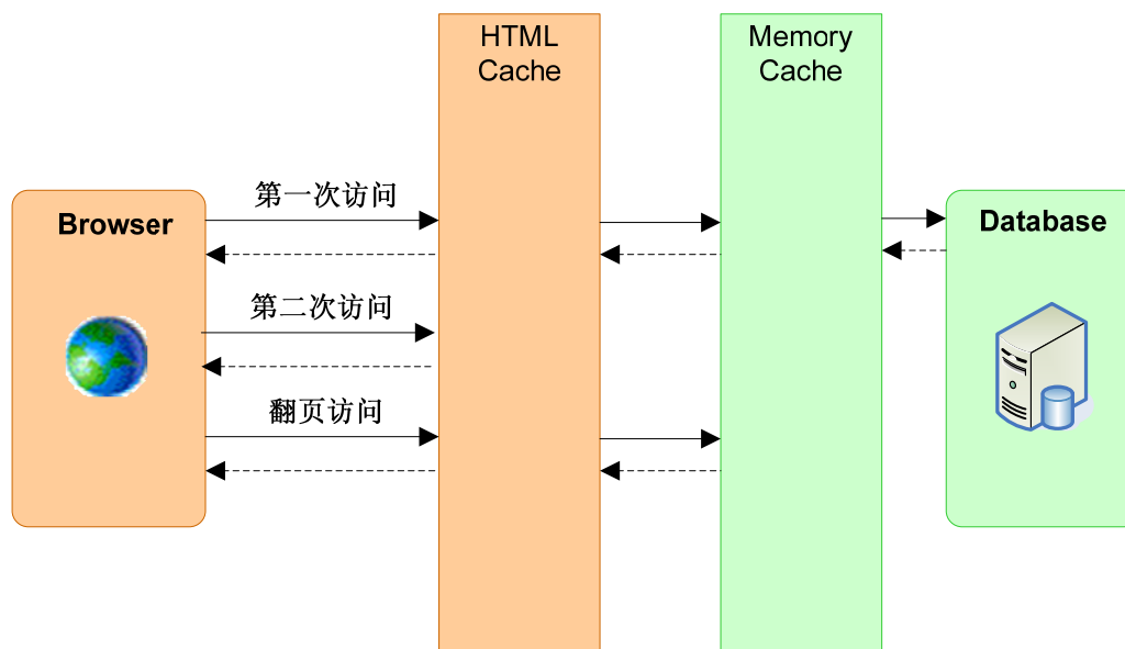
图 5.12 两级缓存实现
