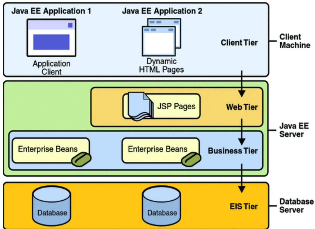
图 2.1 Java EE 体系结构
