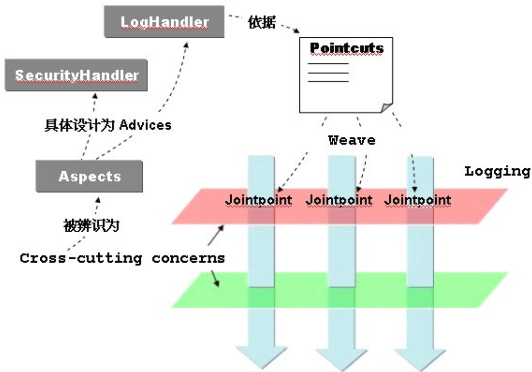
图 2.7 AOP 相关名词示意图
