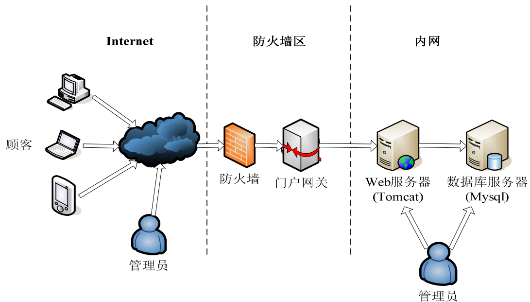
图 6.1 系统网络拓扑图
