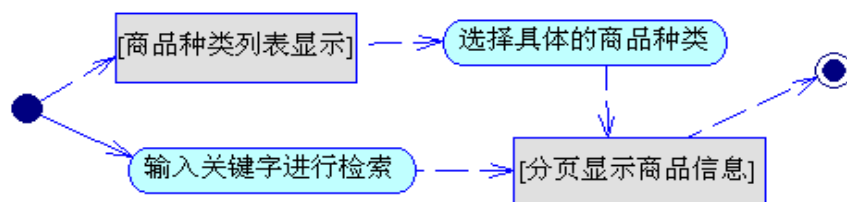
图 5.2 商品检索浏览模块活动图
