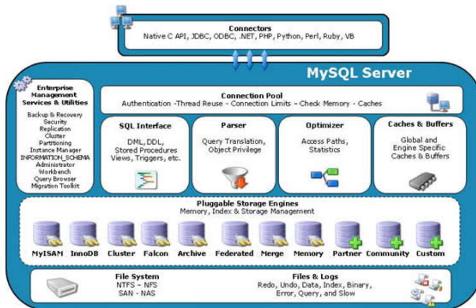
图 2.8 MySQL 数据库架构
