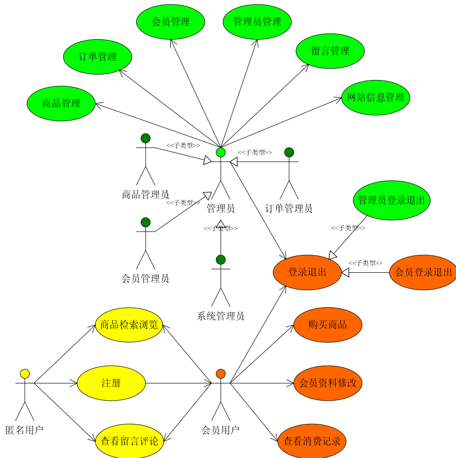
图 4.1 系统主要用例
