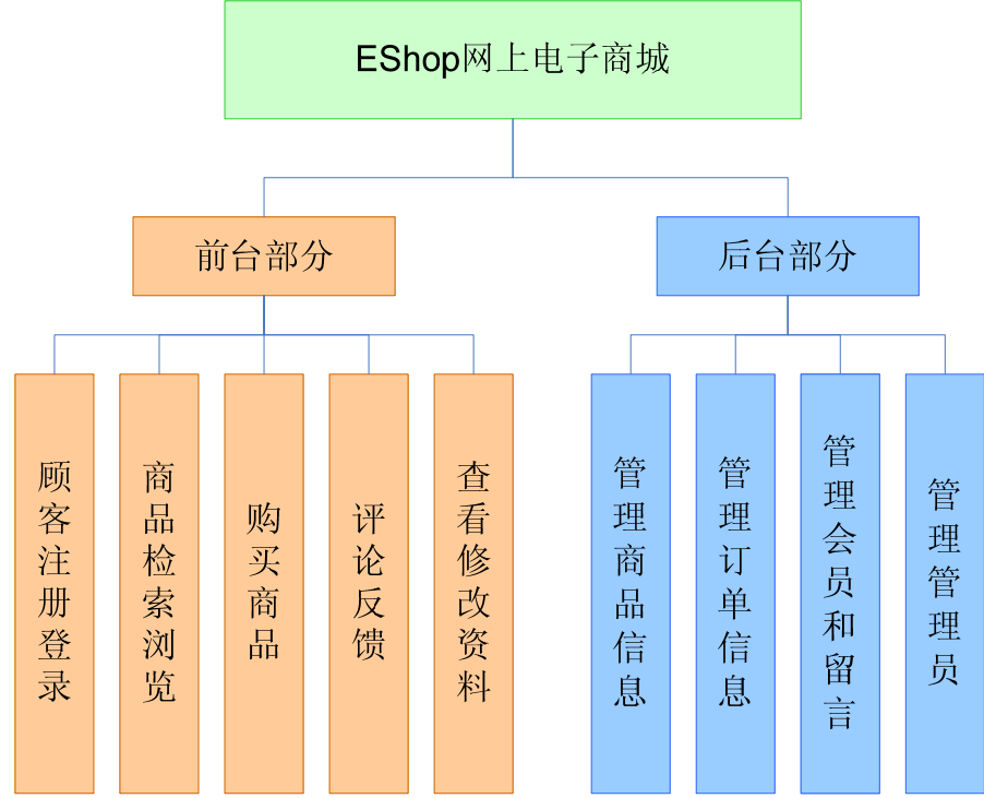
图 3.1 系统具体模块图
