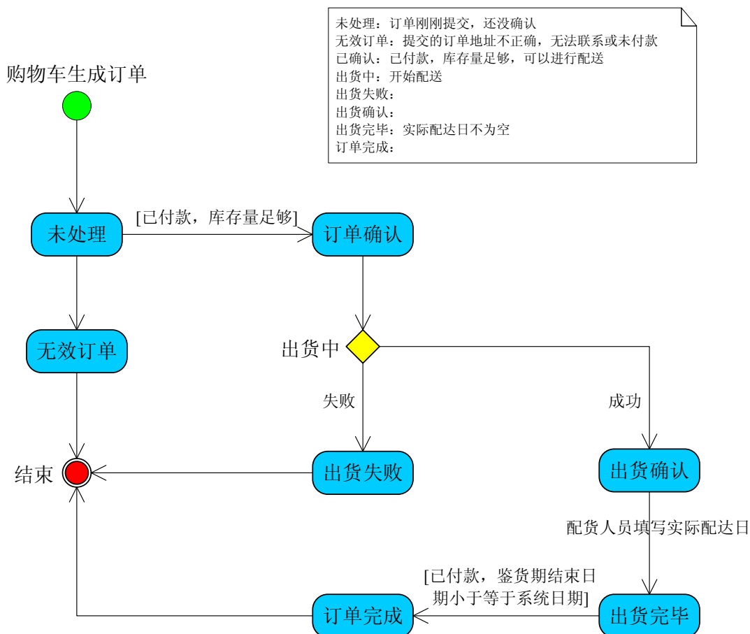
图 4.6 订单状态转换过程
