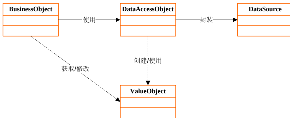
图 2.4 DAO 模式类结构图
