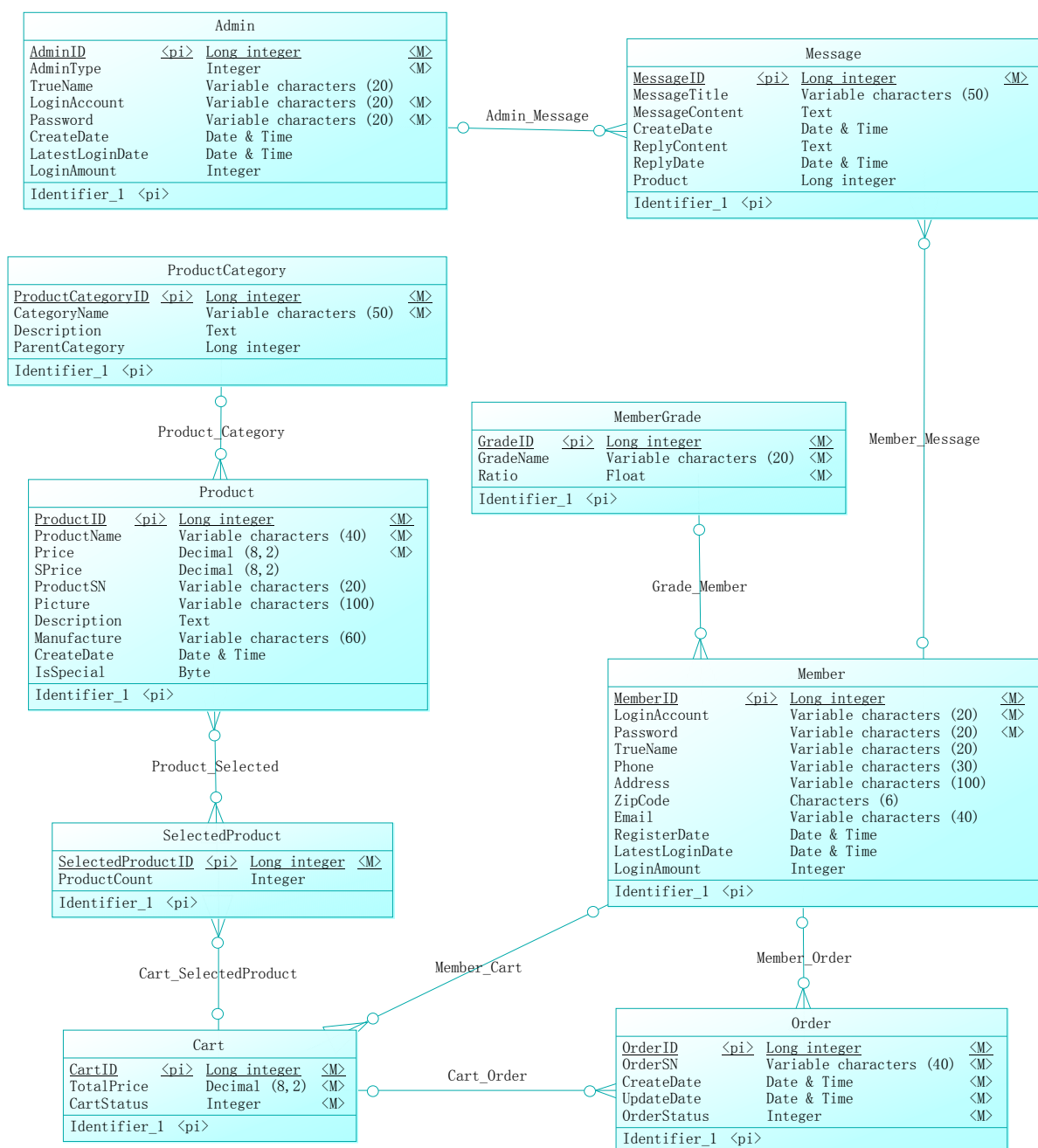
图 5.13 概念数据模型
