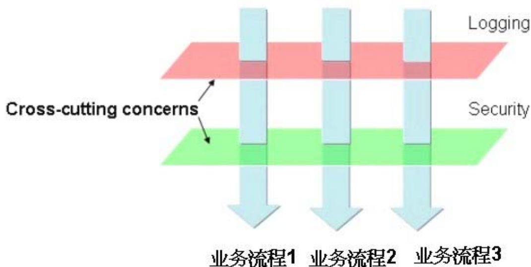
图 2.6 AOP 示意图--Cross-cutting concerns 与业务流程
