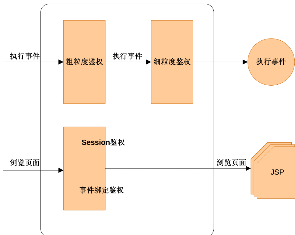
图 5.10 双重权限验证
