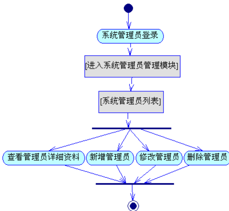
图 5.9 管理员管理模块活动图
