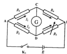
图 3-9-1 电桥原理图
