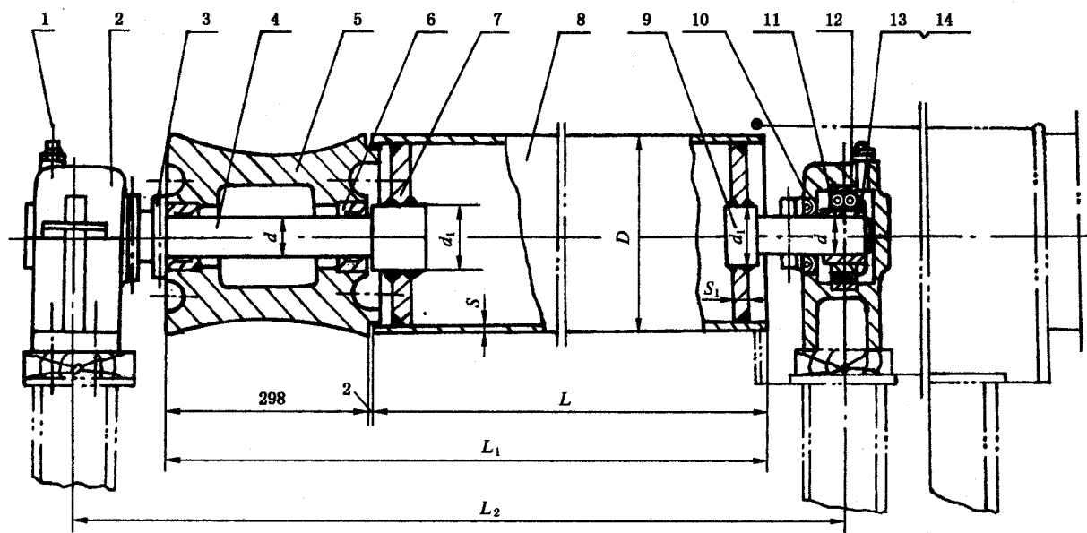
1—油杯;2—轴承座;3—挡圈;4—主长轴;5—摩擦鼓轮;6—衬套;7—端板;8—滚筒体 9—主短轴;10—密封圈;11—紧定套;12—滚动轴承;13—垫片;14—圆螺母
