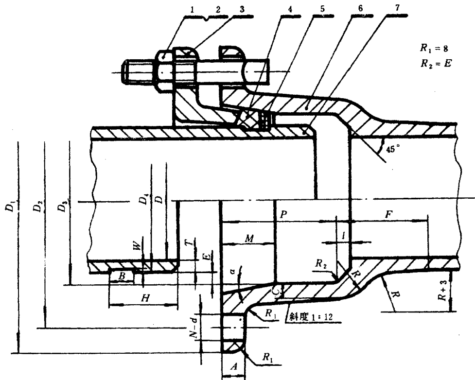
图1 N型胶圈机械接口
