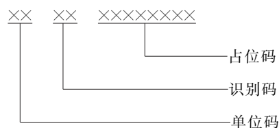
图 1 编码结构图
