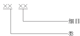
图 1 代码结构图
