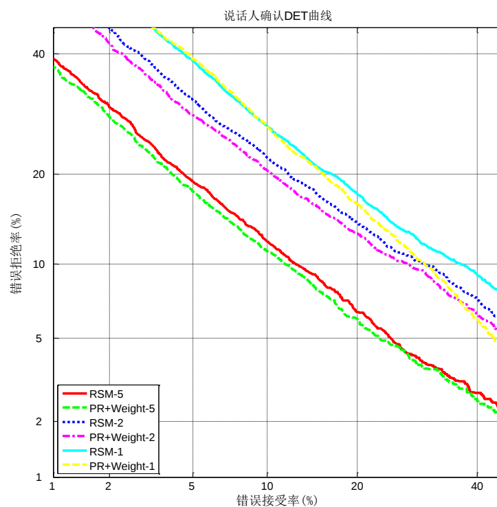
图 3.4 说话人确认 DET 曲线
