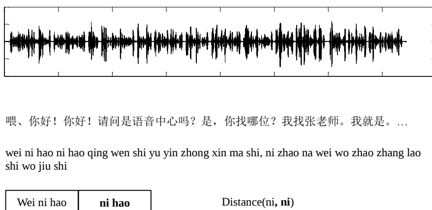
图 3.1 基于音素识别和文本相关的说话人分割算法示意图
