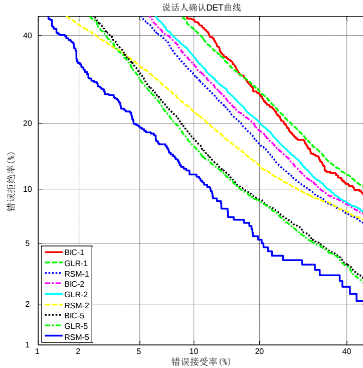
图 2.5 短语音说话人确认性能比较实验
