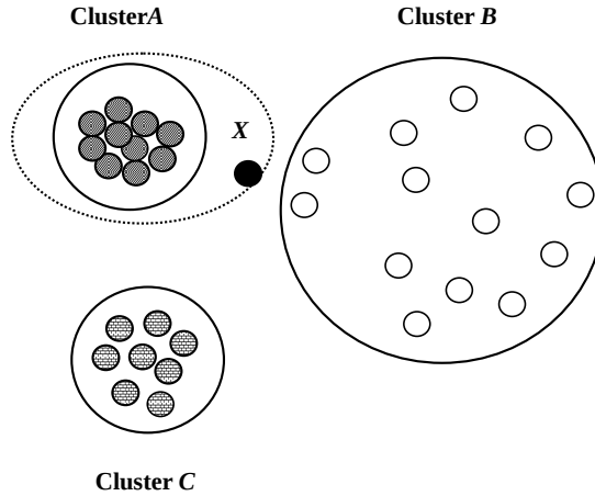
图 4.2 HAC 算法合并示意图
