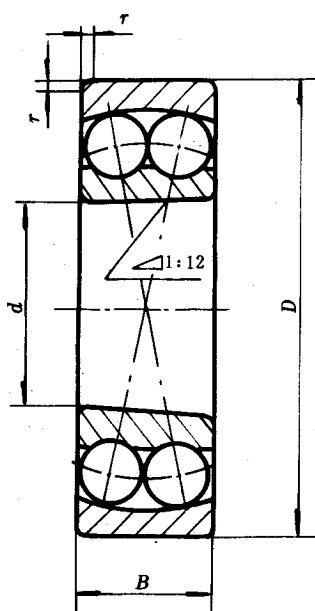
图 2 圆锥孔调心球轴承 10000 K 型
