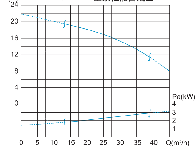
50WQ/S202-3型泵主要参数
