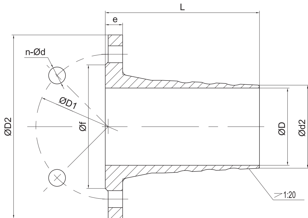
软管直接头
