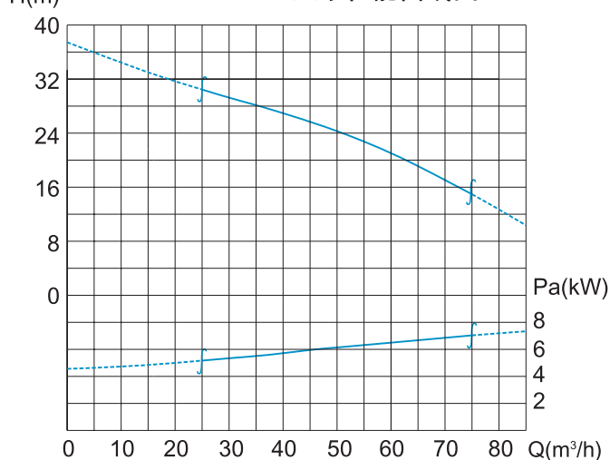
65WQ/S205-7.5型泵性能曲线图
