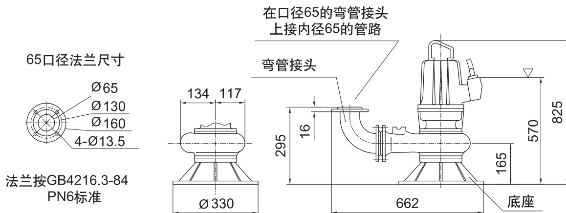
65WQ/S205-7.5型泵 第2种接硬管的立式底座安装尺寸图
