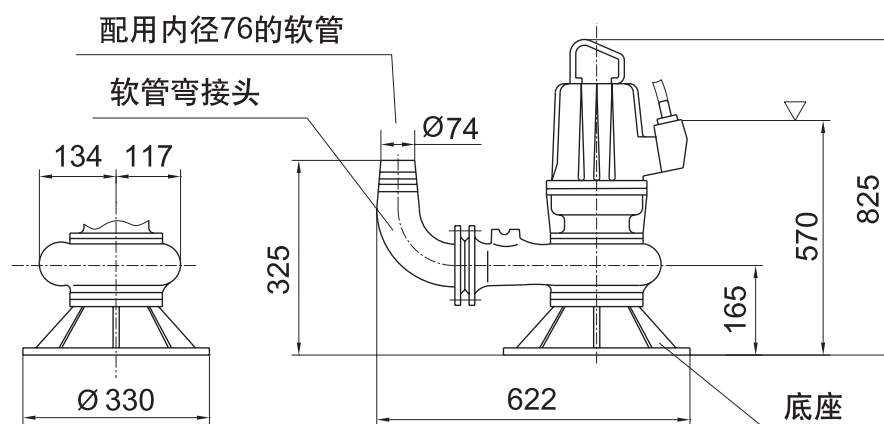
LR 65WQ/S205-7.5型泵 接软管的立式底座安装尺寸图
