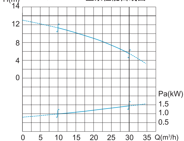
50WQ/S402-1.5型泵主要参数
