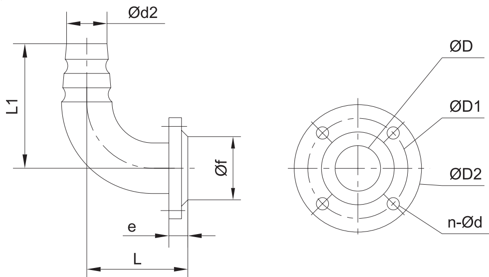
软管弯接头
