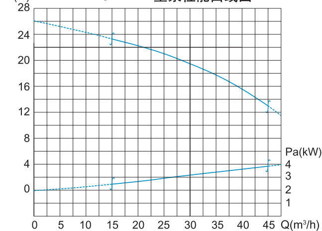
50WQ/S201-4型泵主要参数
