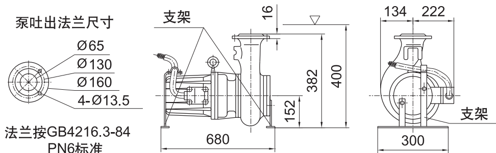
65WQ/S205-7.5型泵 第2种接硬管的卧式支架安装尺寸图
