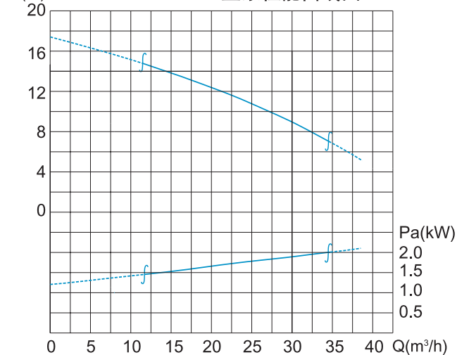
50WQ/S401-2.2型泵主要参数
