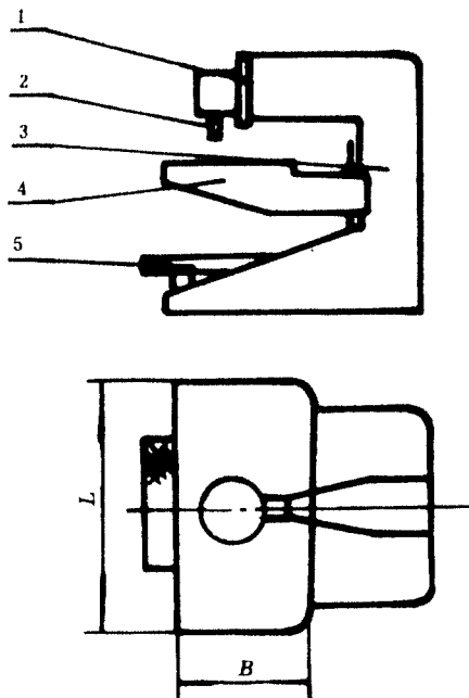
1—主轴滑座；2—主轴；3—床身； 4—工作台；5—脚踏装置
