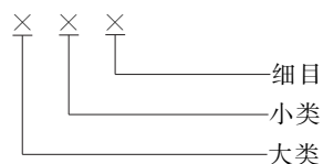
图 1 代码结构图
