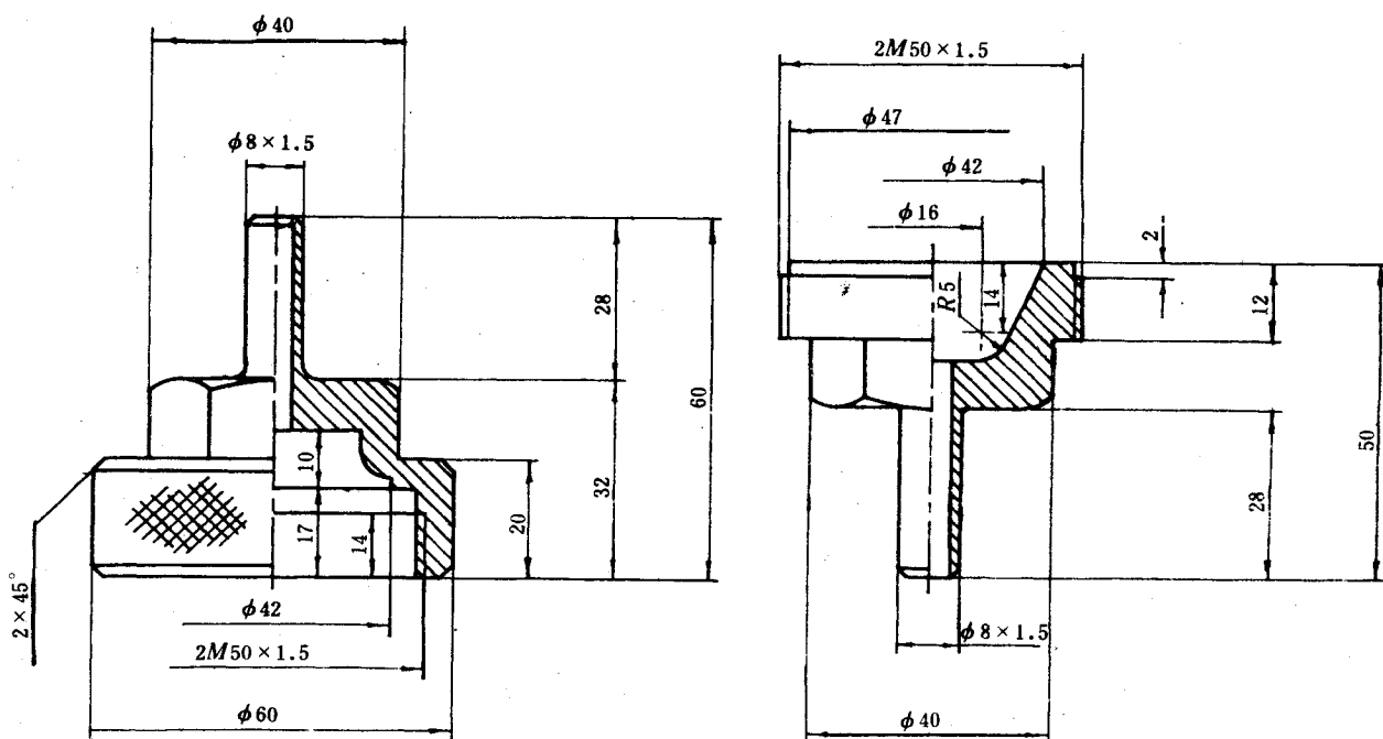
图1 取样器（尼龙）
