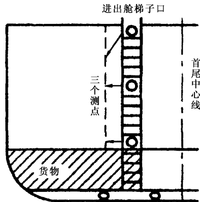
图 1 货舱盖未打开时人孔内采样点位置
