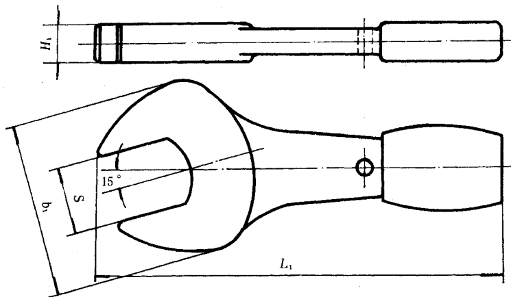
图 1 敲击呆扳手
