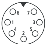
位置测量系统 (数字输出) 元件插头 (对着极柱端面看)
