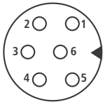
位置测量系统 (模拟输出) 元件插头 (对着极柱端面看)
