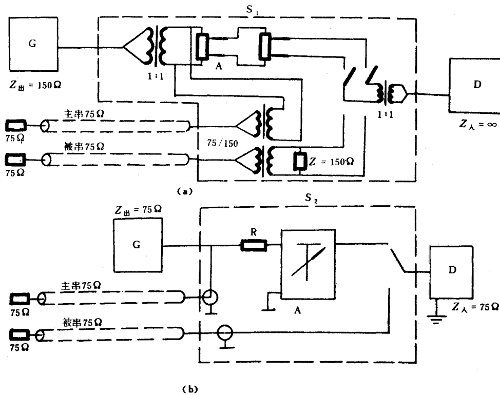
图1 同轴对之间的近端串音衰减 (简称同串同)
