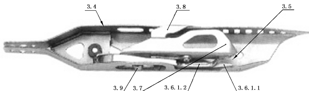
图1 送纬剑头
