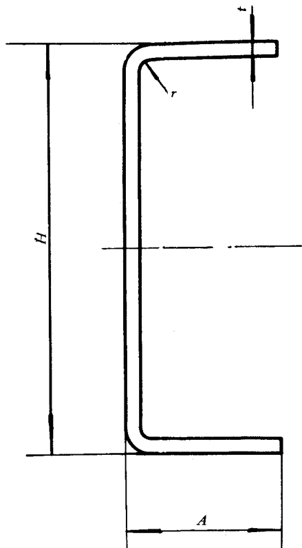
图 1 槽形型钢
