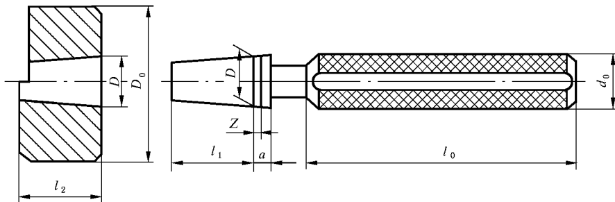
图 1 钻夹圆锥量规型式
