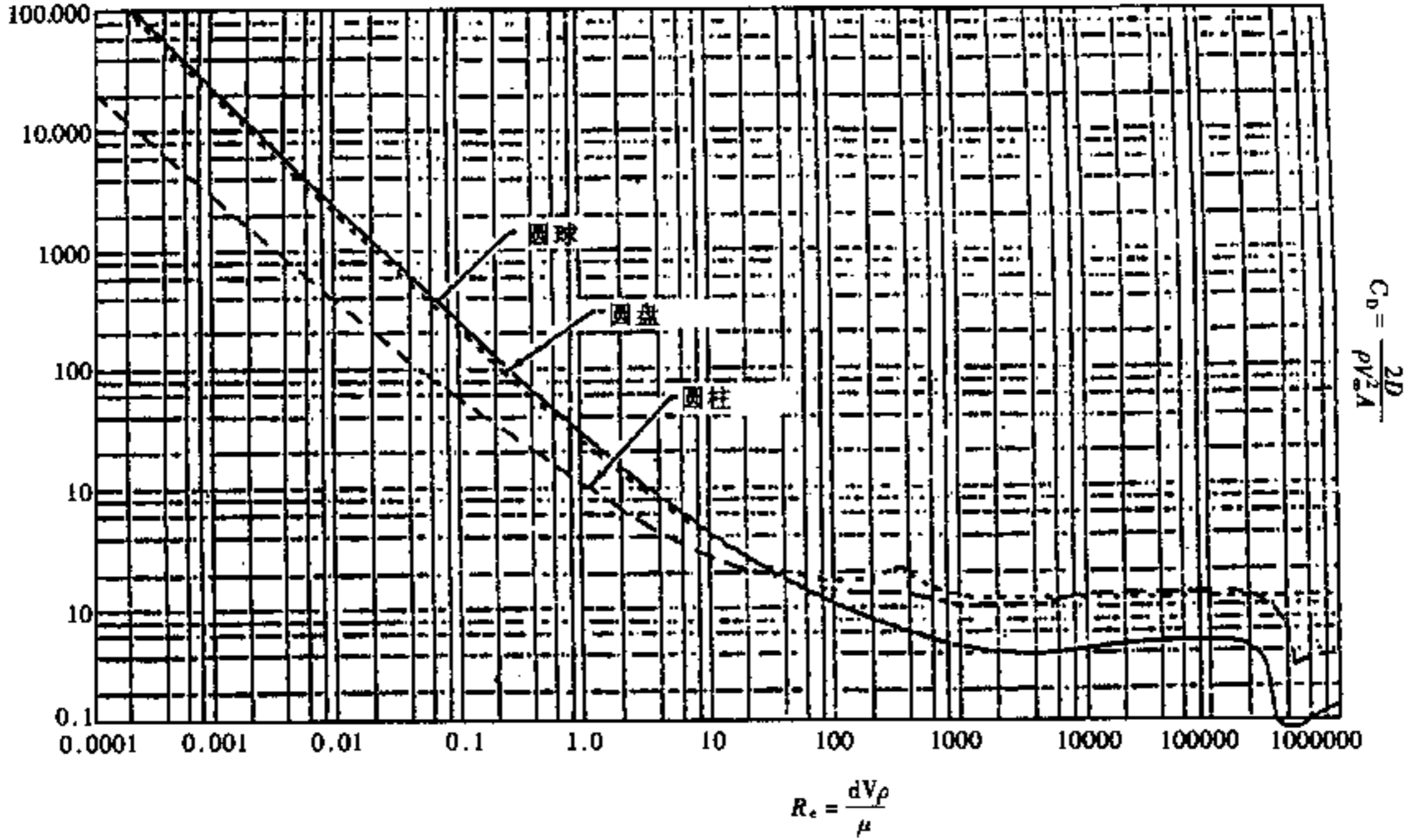
C_D - R_e 曲线
