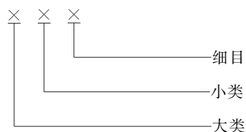
图 1 代码结构图
