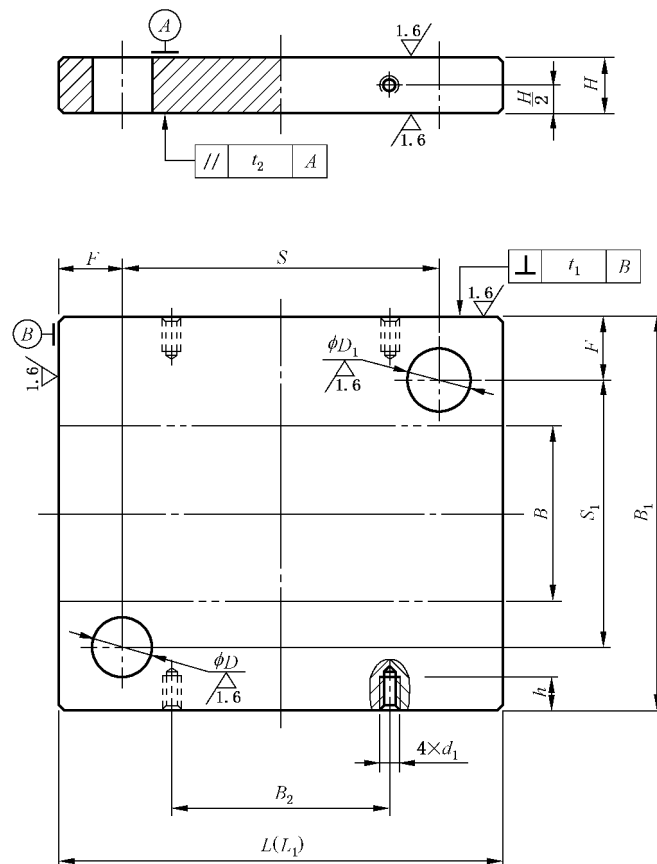
图 1 滑动导向对角导柱上模座
