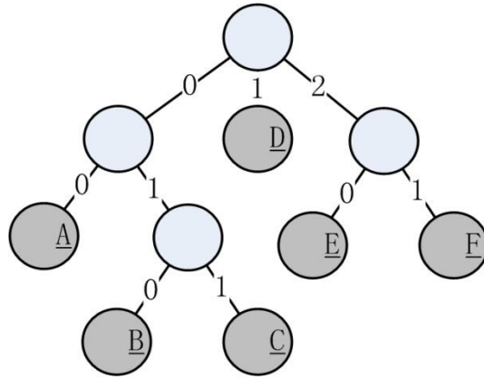
图 6.4 逻辑子句绝对位置模式标记
