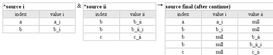
图 5.2 集合数据源接续算法机制示意图
