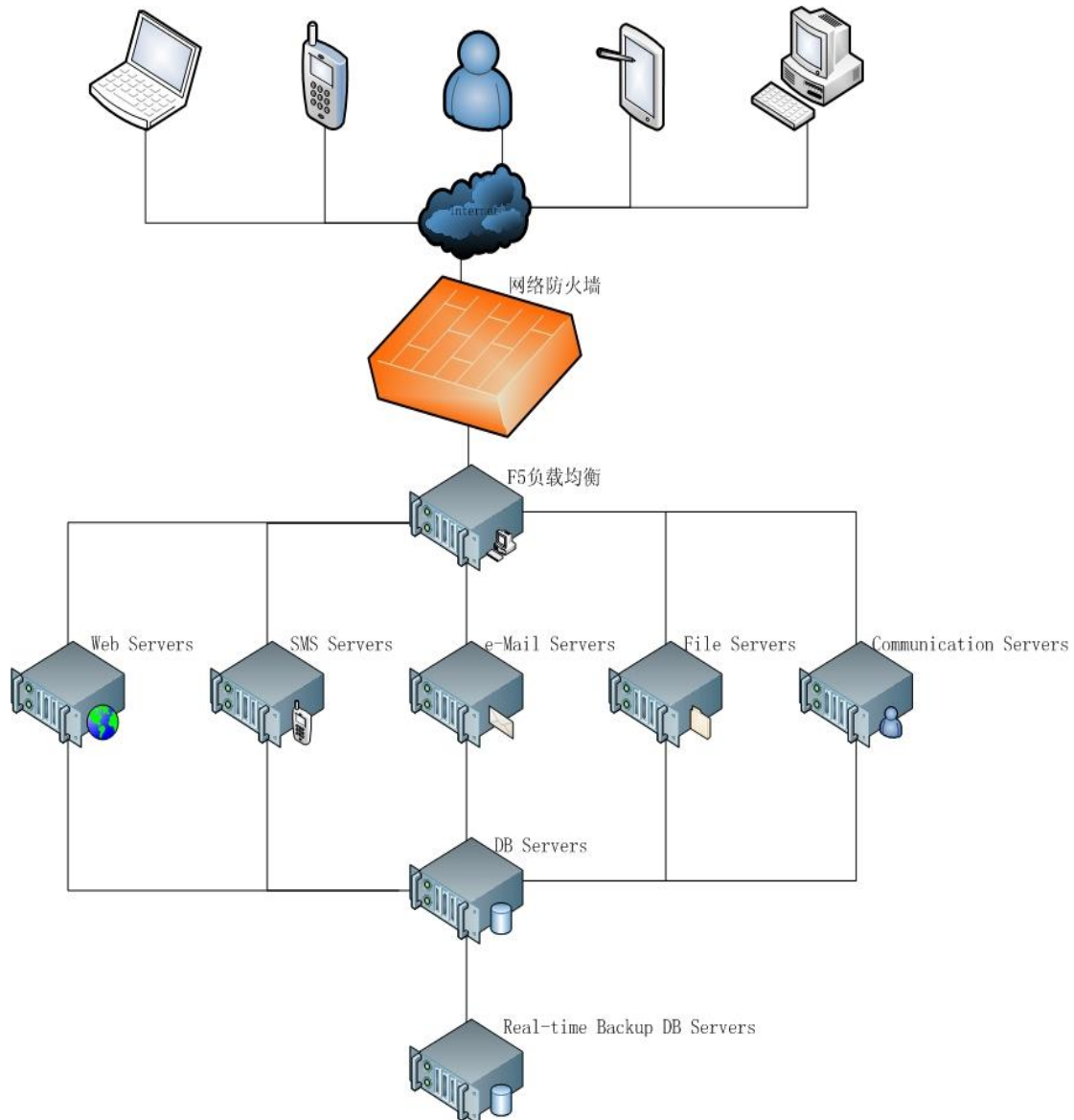
图 3.1 系统架构图
