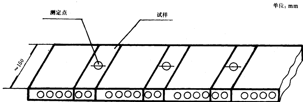
图 1 在全厚度样品测定点切取的试样
