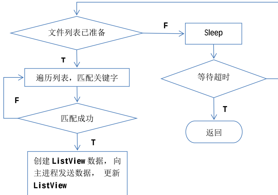
图 3.18 文件搜索流程图
