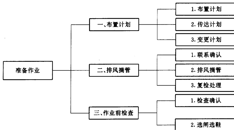
图 1 铁路调车准备作业程序图
