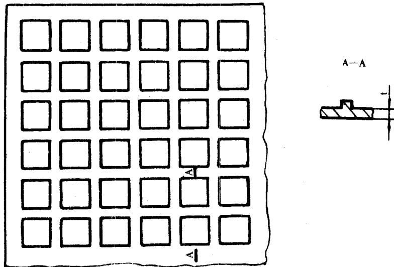
图 1 1号花纹板
