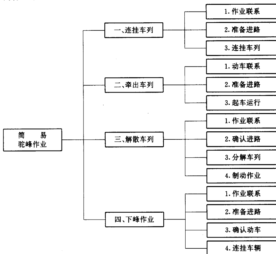
图1 铁路调车简易驼峰作业程序图
